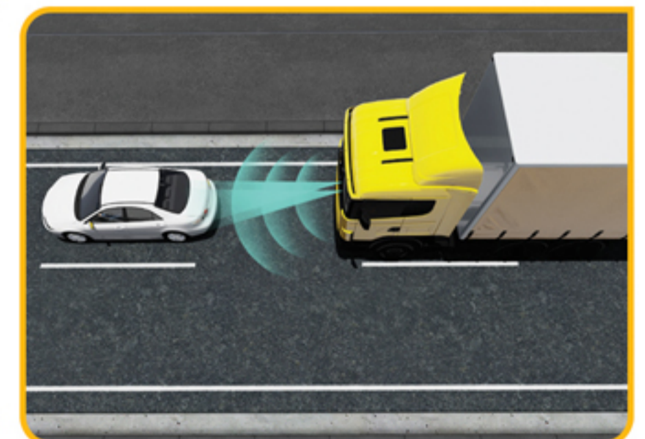
کروز کنترل تطبیقی (ACC)
